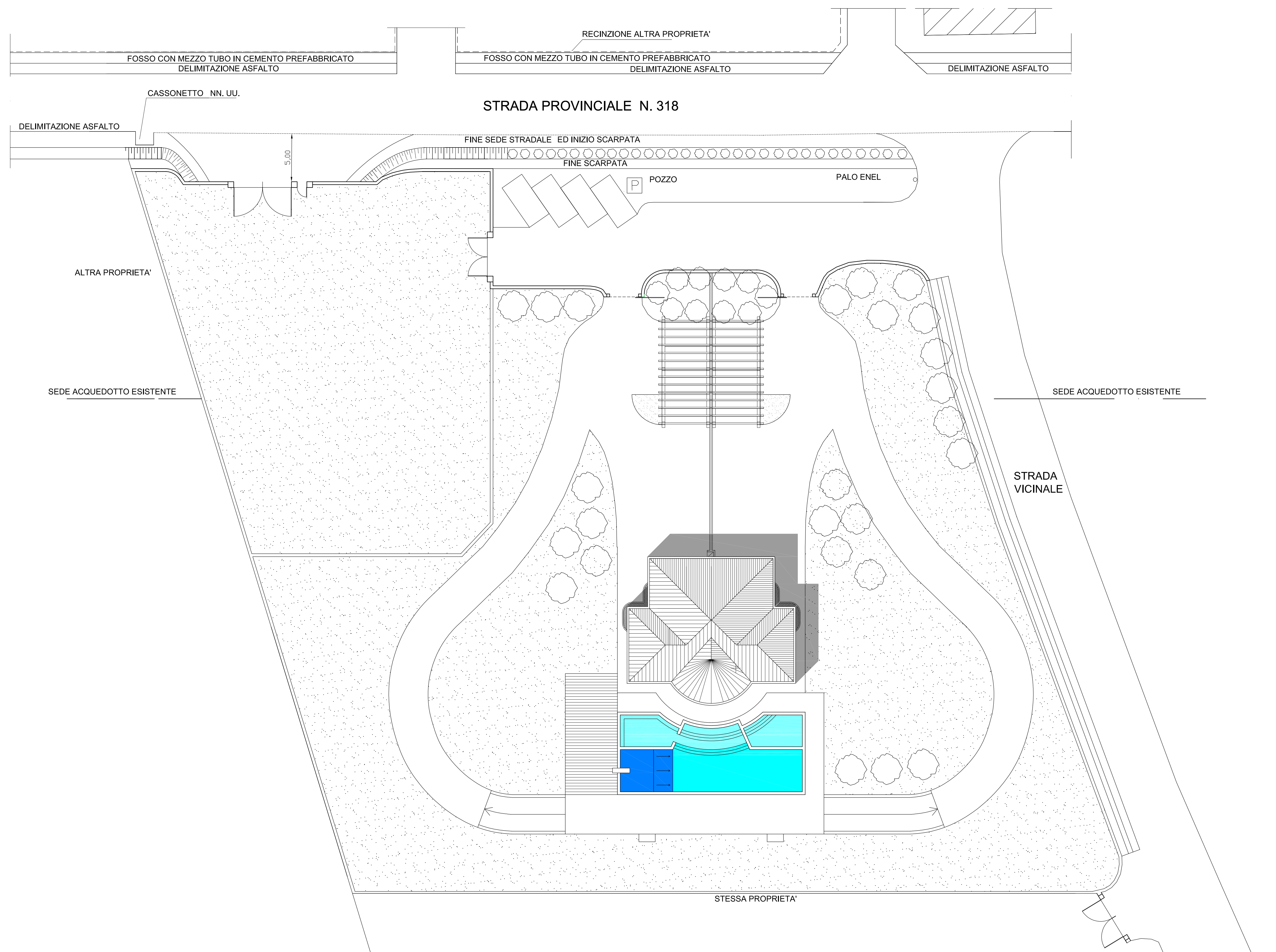
PLANIMETRIA GENERALE - STATO VARIATO - SCALA 1 : 200
